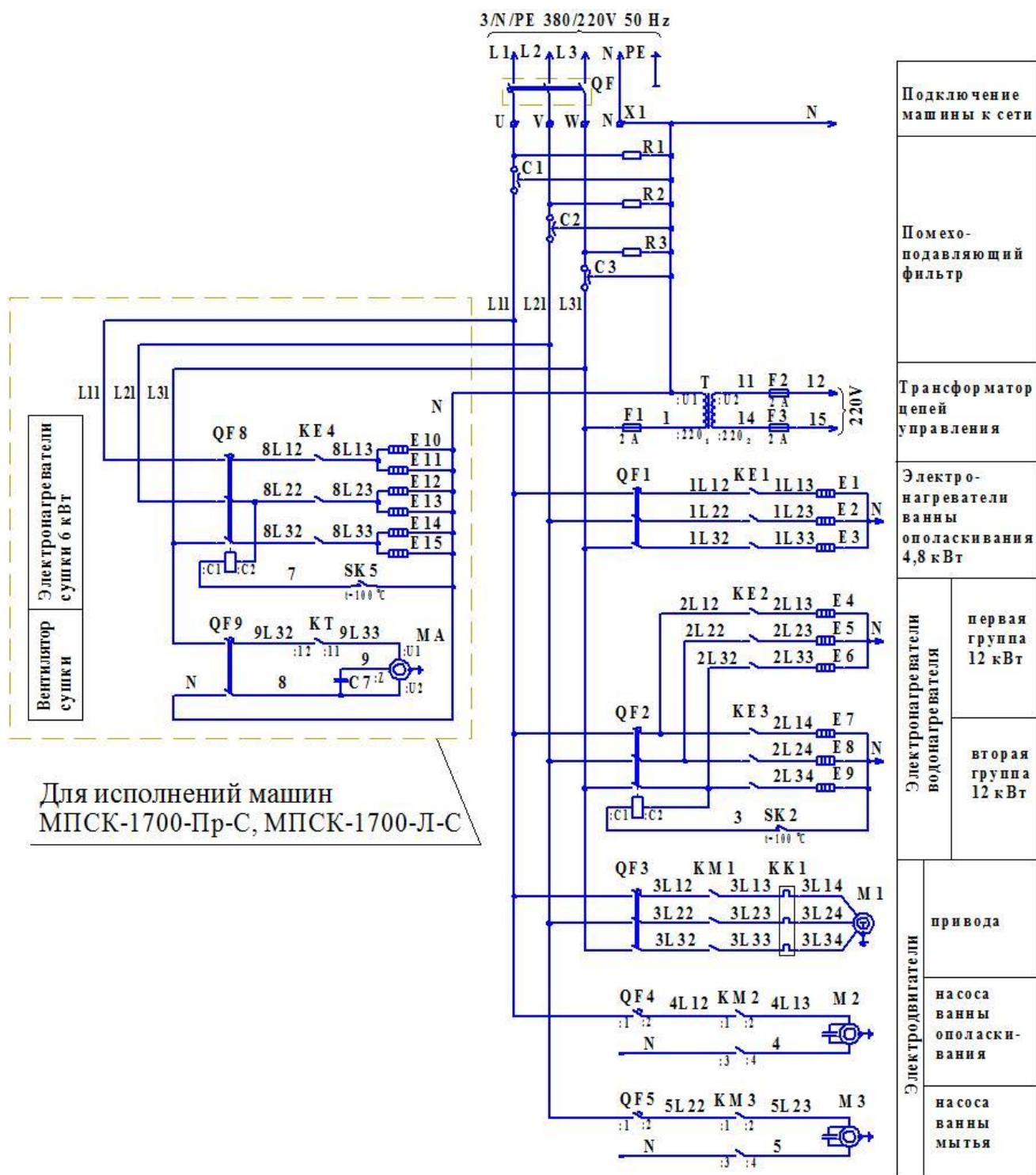
Рисунок 3 (лист 1 из 2) - Схема электрическая принципиальная машин МПСК
