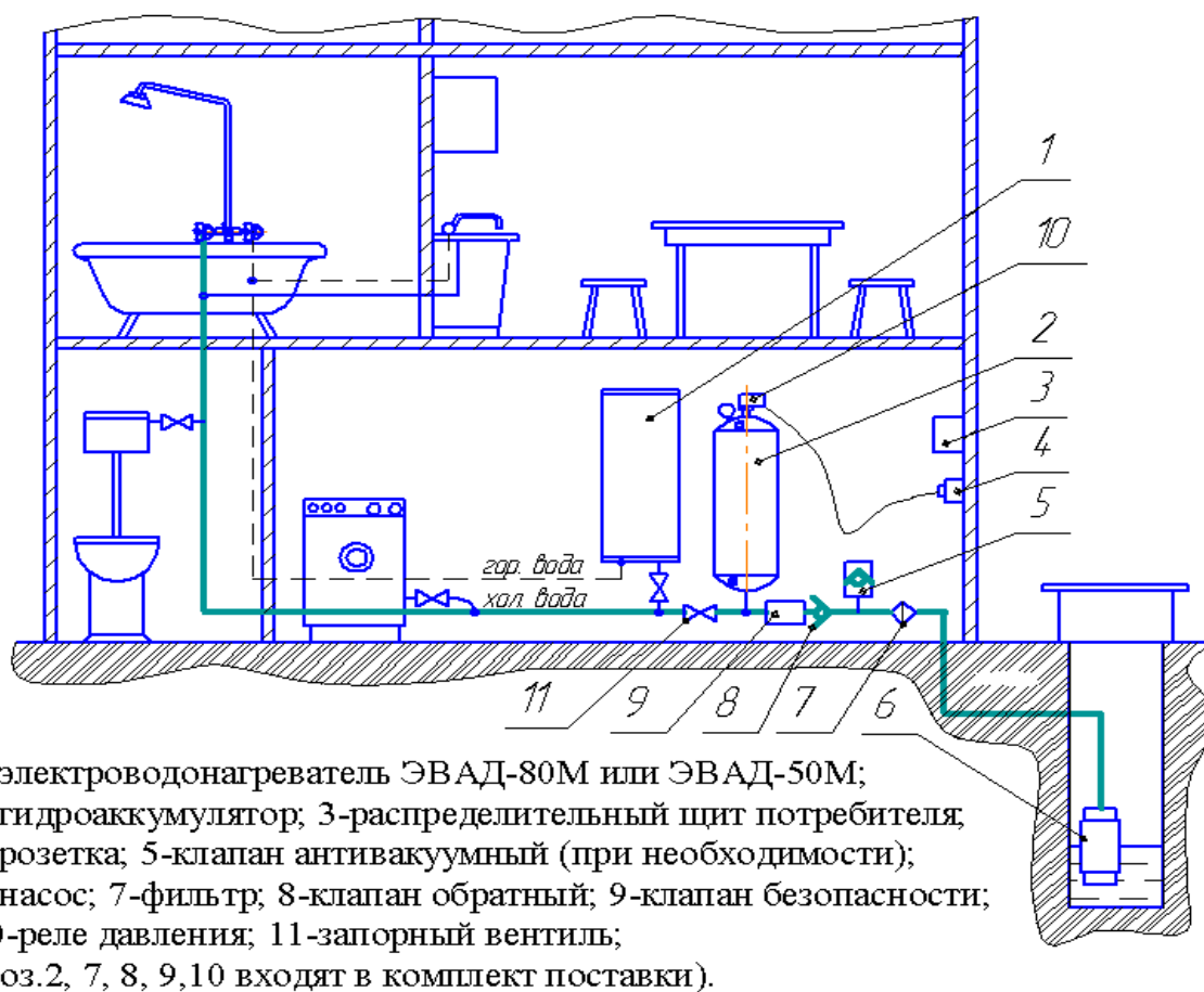
Рисунок 3 – Схема подключения гидроаккумулятора к водопроводным сетям жилого дома
